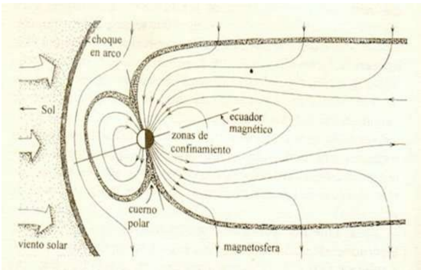
Figura 7.1 . El campo magnético de la Tierra, confinado por el viento solar en una cavidad con forma de cometa denominada magnetósfera. El viento comprime la magnetosfera del lado del día en una capa de unos 10 radios terrestres aproximadamente. En el lado de la noche, el viento "barre" ese campo magnético, convirtiéndolo en una "cola magnética" de como mínimo 1000 radios
